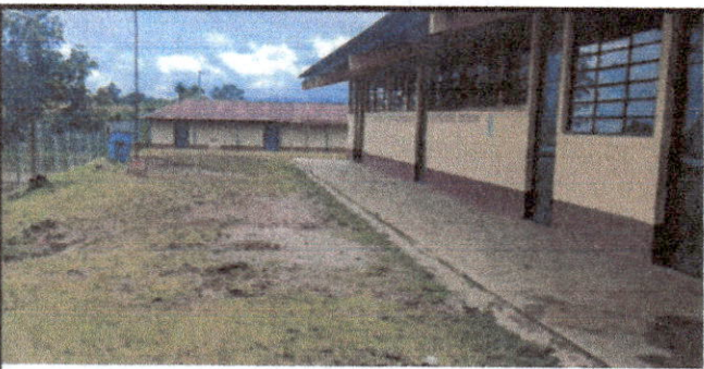
Foto 5: Reparación de planchas de concreto de patio
