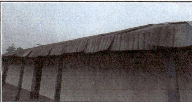
Foto 1: Sustrucción de lamina por lamina troquelada aluzinc calibre 26
